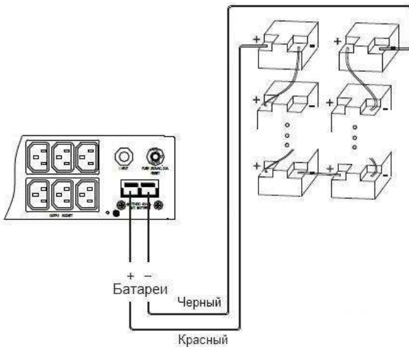
Схема подклюочения внешних батарей для ИБП 1кВА - 3кВА
