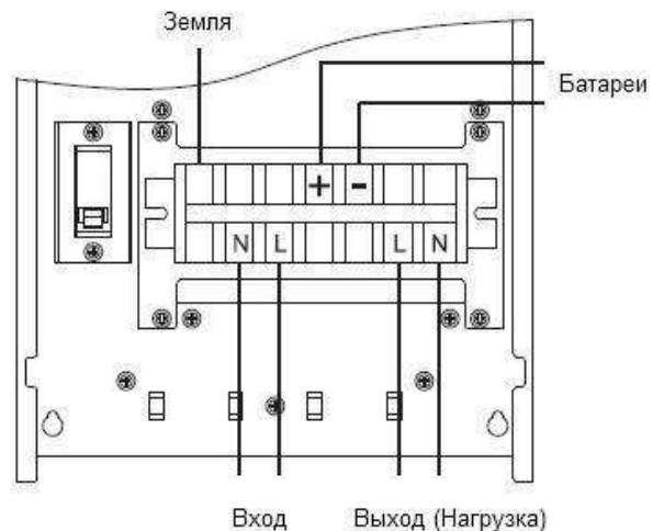
Схема подключения для моделей 6кВа и 10кВа
