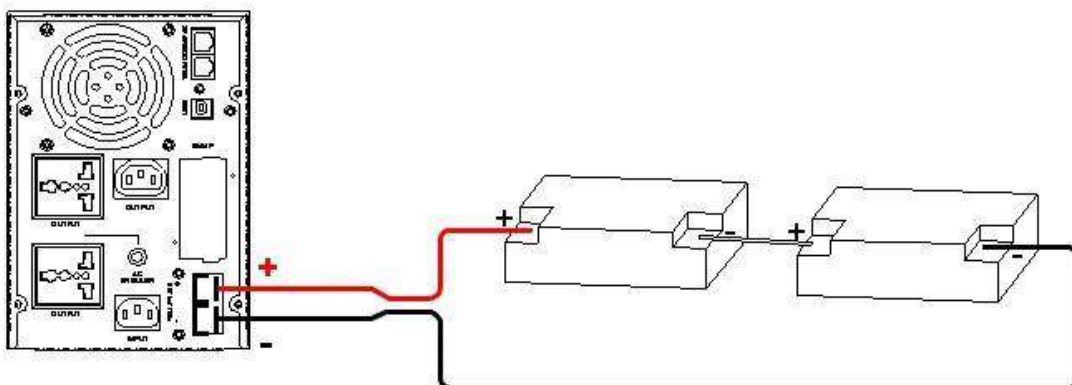
Корпус Tower. Схема подключения аккумуляторных батарей Напряжение постоянного тока U=24V .
