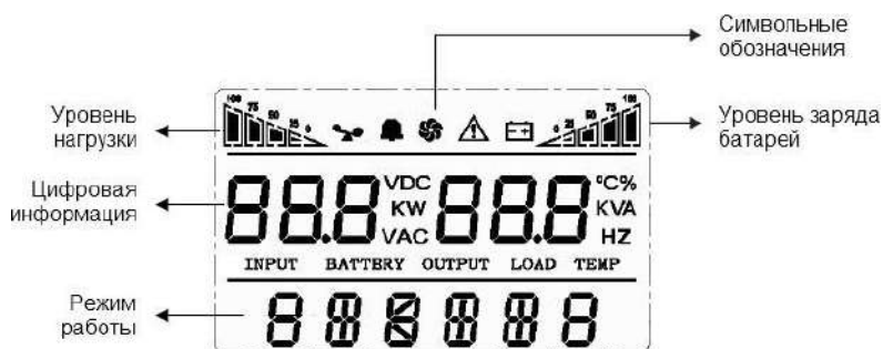
LCD-дисплей. Корпус Tower.
