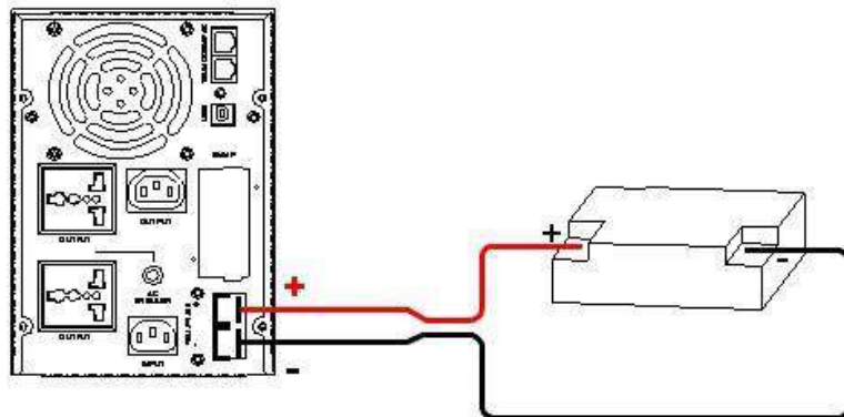
Корпус Tower. Схема подключения аккумуляторных батарей. Напряжение постоянного тока U=12V .
