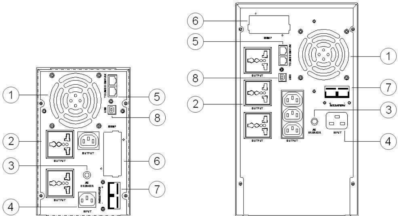
Корпус Tower. Задняя панель ИБП 500 ВА – 2 кВА
