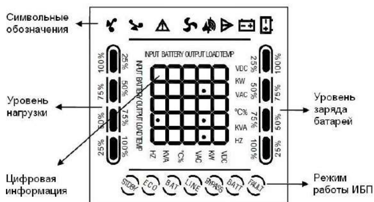
LCD-дисплей. Корпус Rack Tower.
